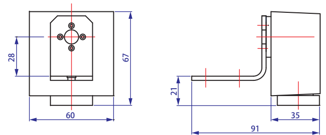
リモコン雲台外形寸法
